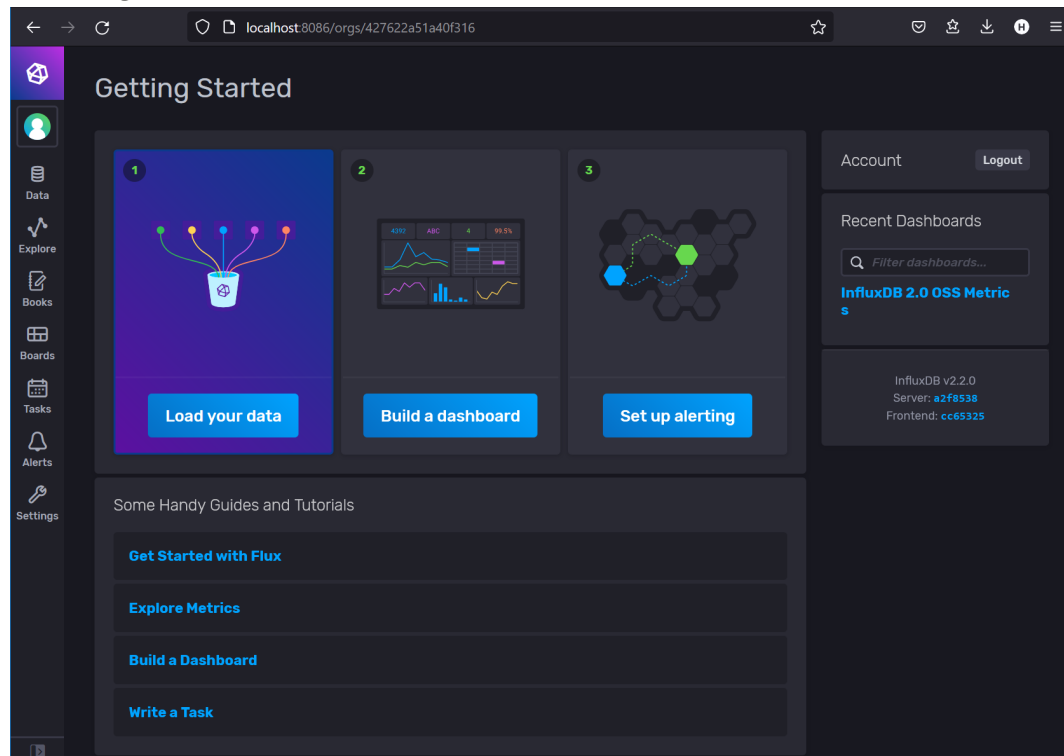
Abbildung 2: InfluxDB Dashboard
